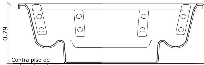
CORTE A A SPA EXTERNO
