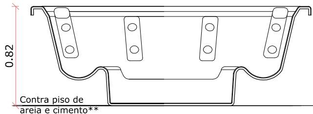
CORTE A A SPA EXTERNO
