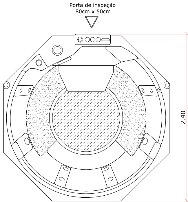
PLANTA BAIXA
