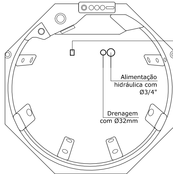
PLANTA HIDÁULICA E ELÉTRICA
