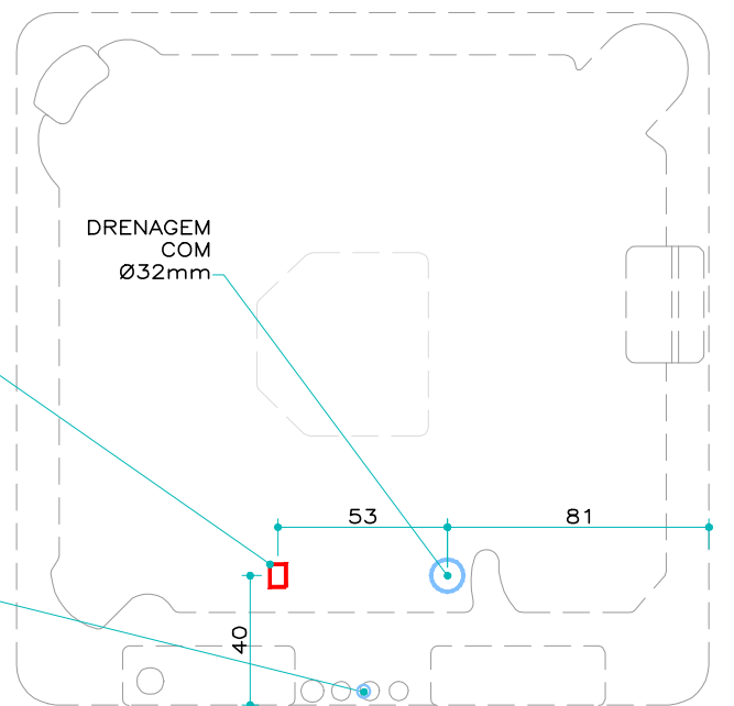
SPA EXTERNO ESCALA 1:25
