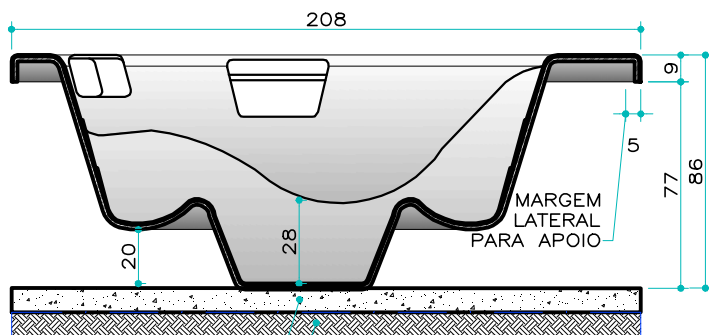
CONTRAPISO DE AREIA E CIMENTO** TERRENO BEM APOIADO
